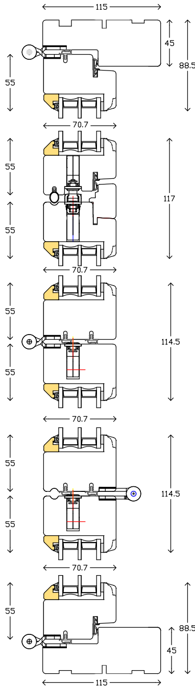
Vandret snit
