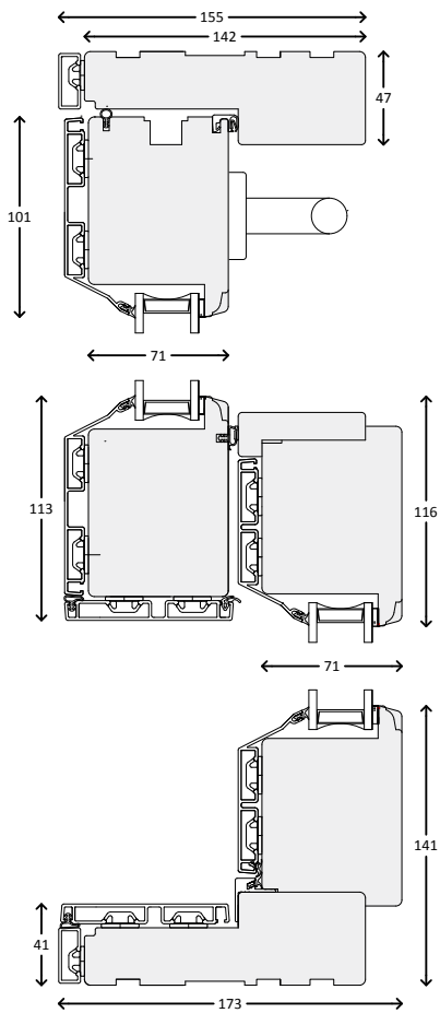
Vandret snit
