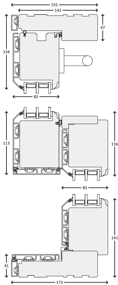
Vandret snit
