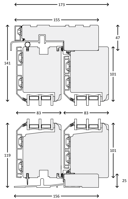
Lodret snit
