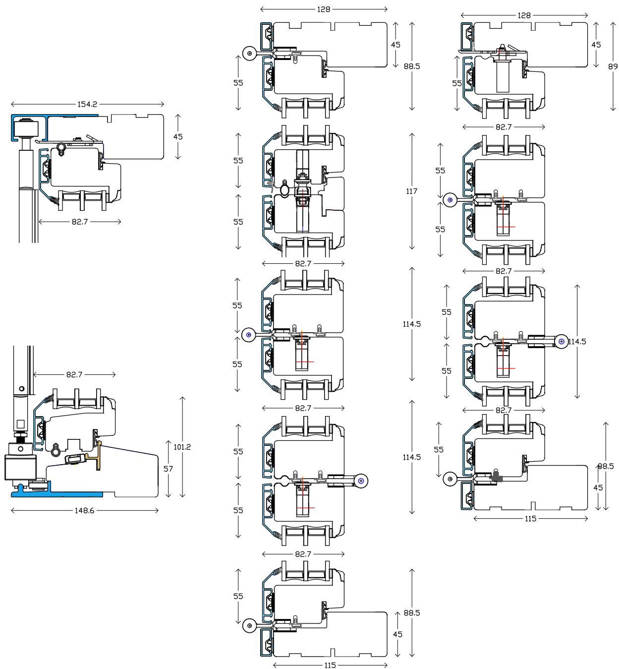
Lodret snit
