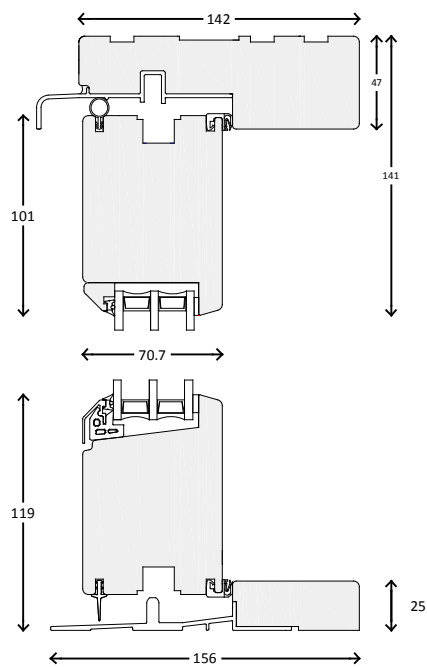
Lodret snit - Gående ramme
