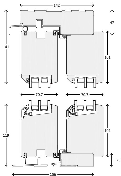
Lodret snit - Stående ramme
