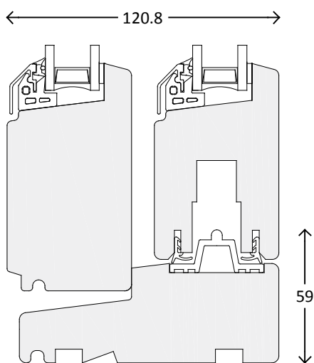
Lodret snit
