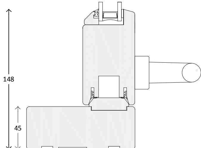
Vandret snit
