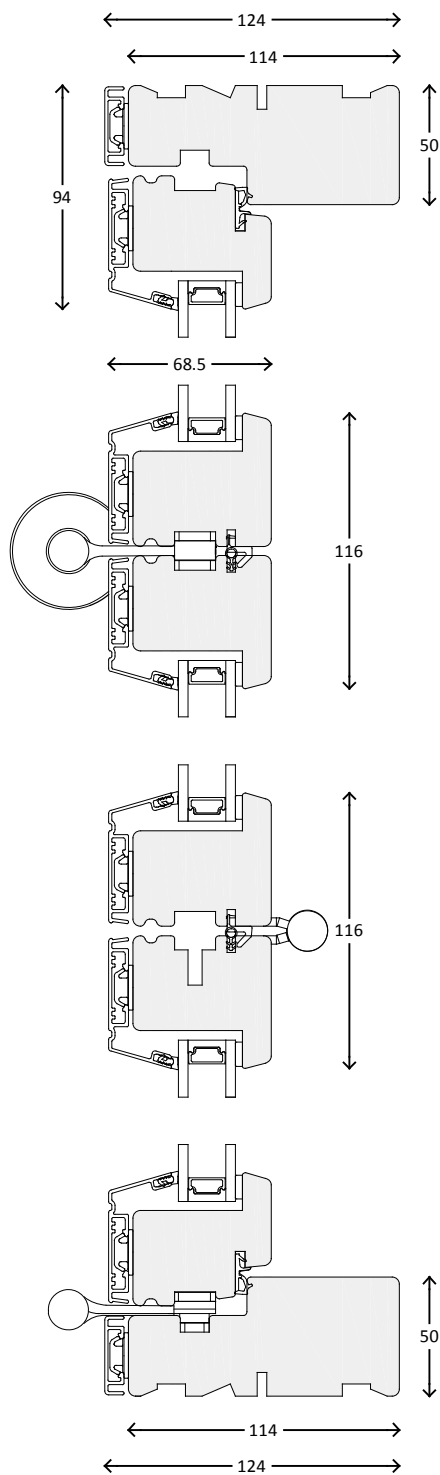
Vandret snit
