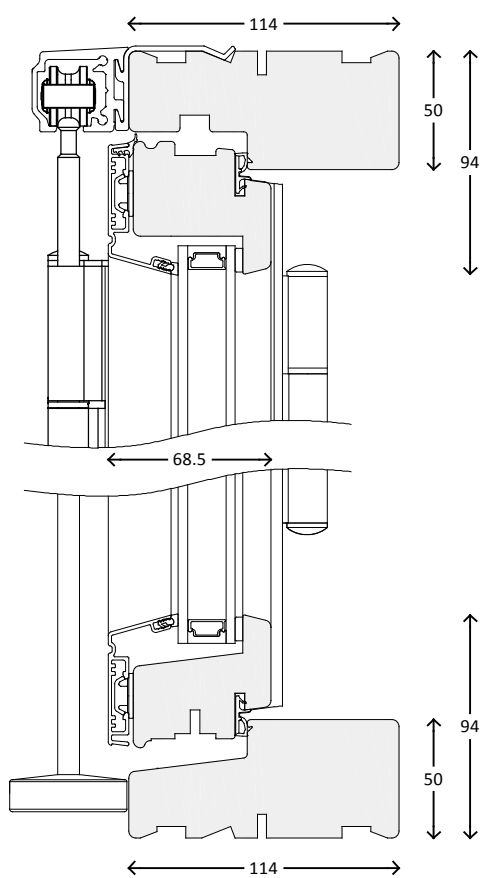
Lodret snit
