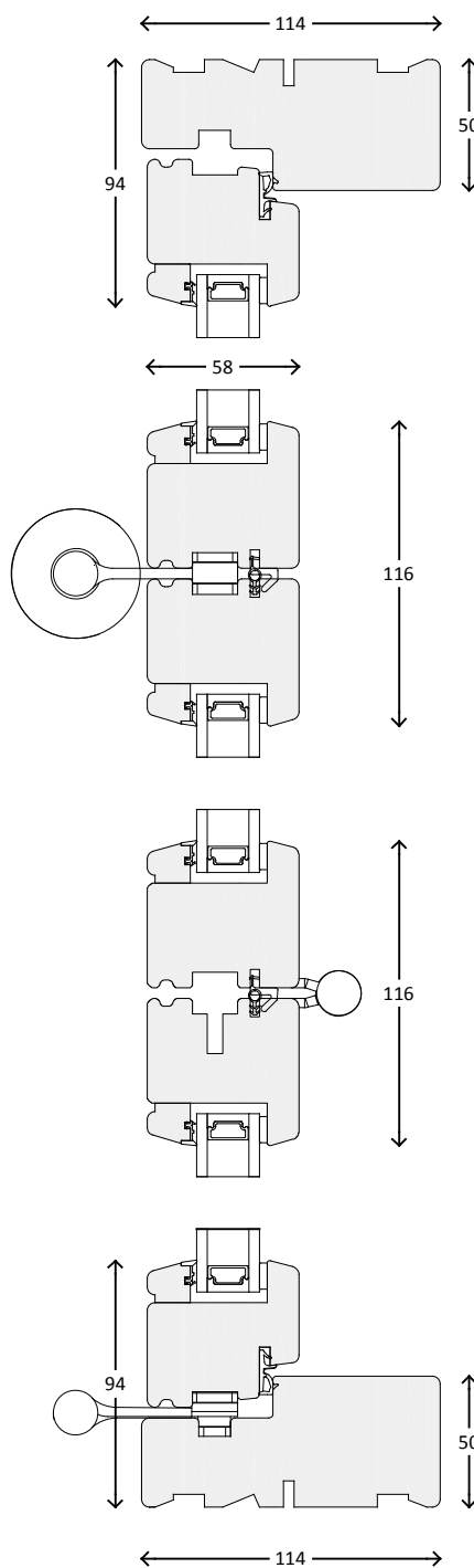
Vandret snit
