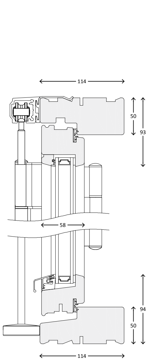
Lodret snit
