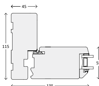
Sidekarm
