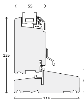
Bundkarm hårdtræ
