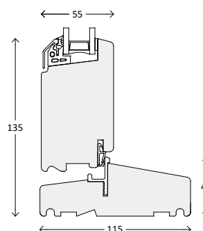
Bundkarm hårdtræ
