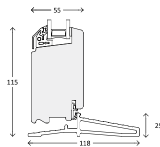
Bundkarm Komposit
