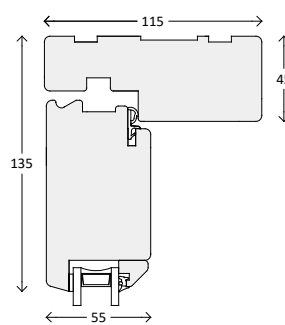
Overkarm
