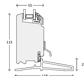
Bundkarm Komposit
