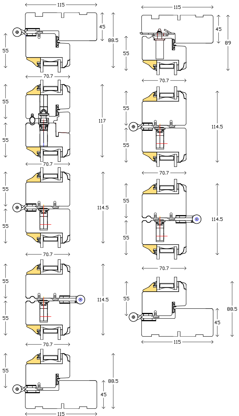
Vandret snit
